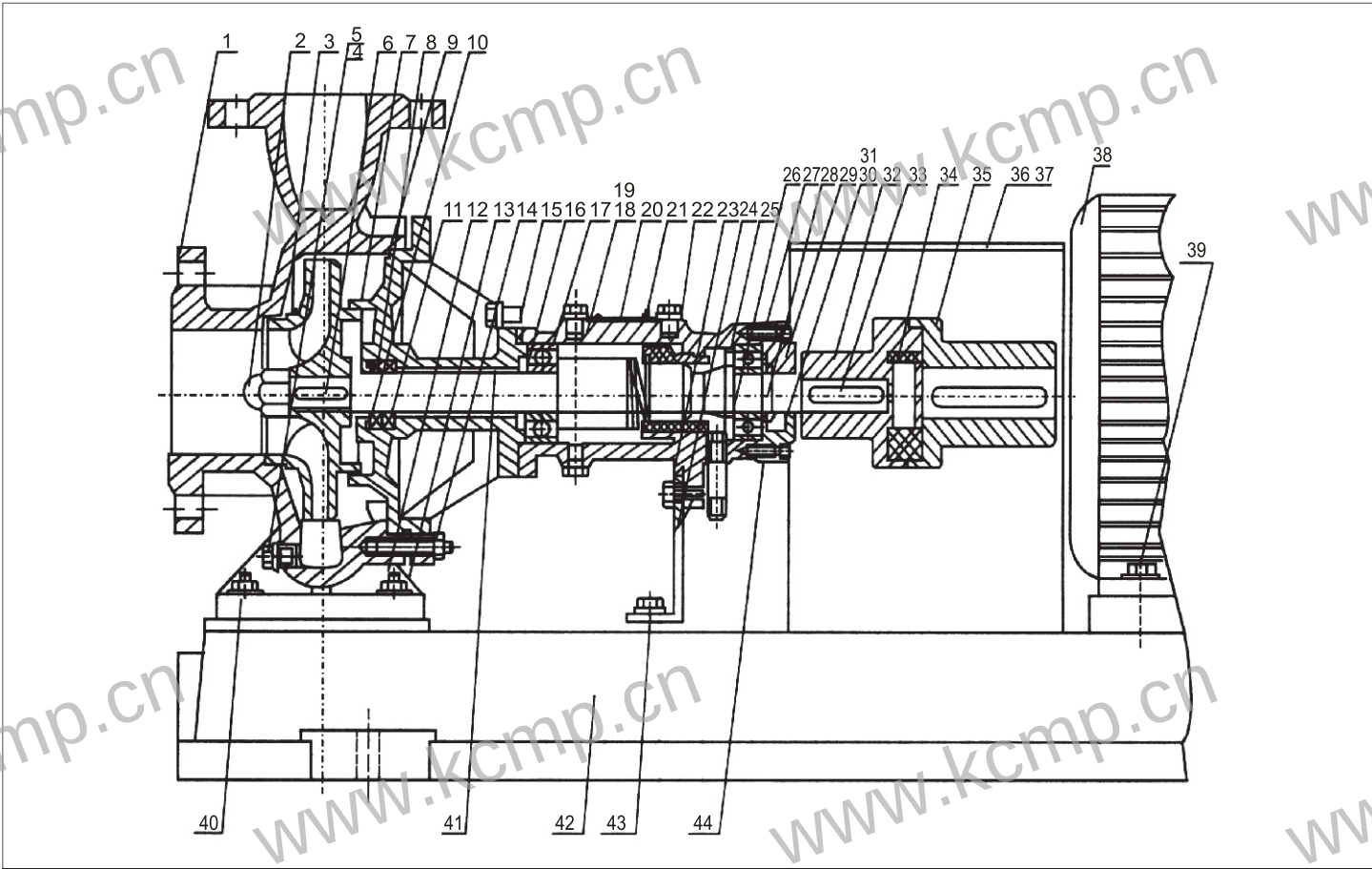
结构图 Structural Drawing
