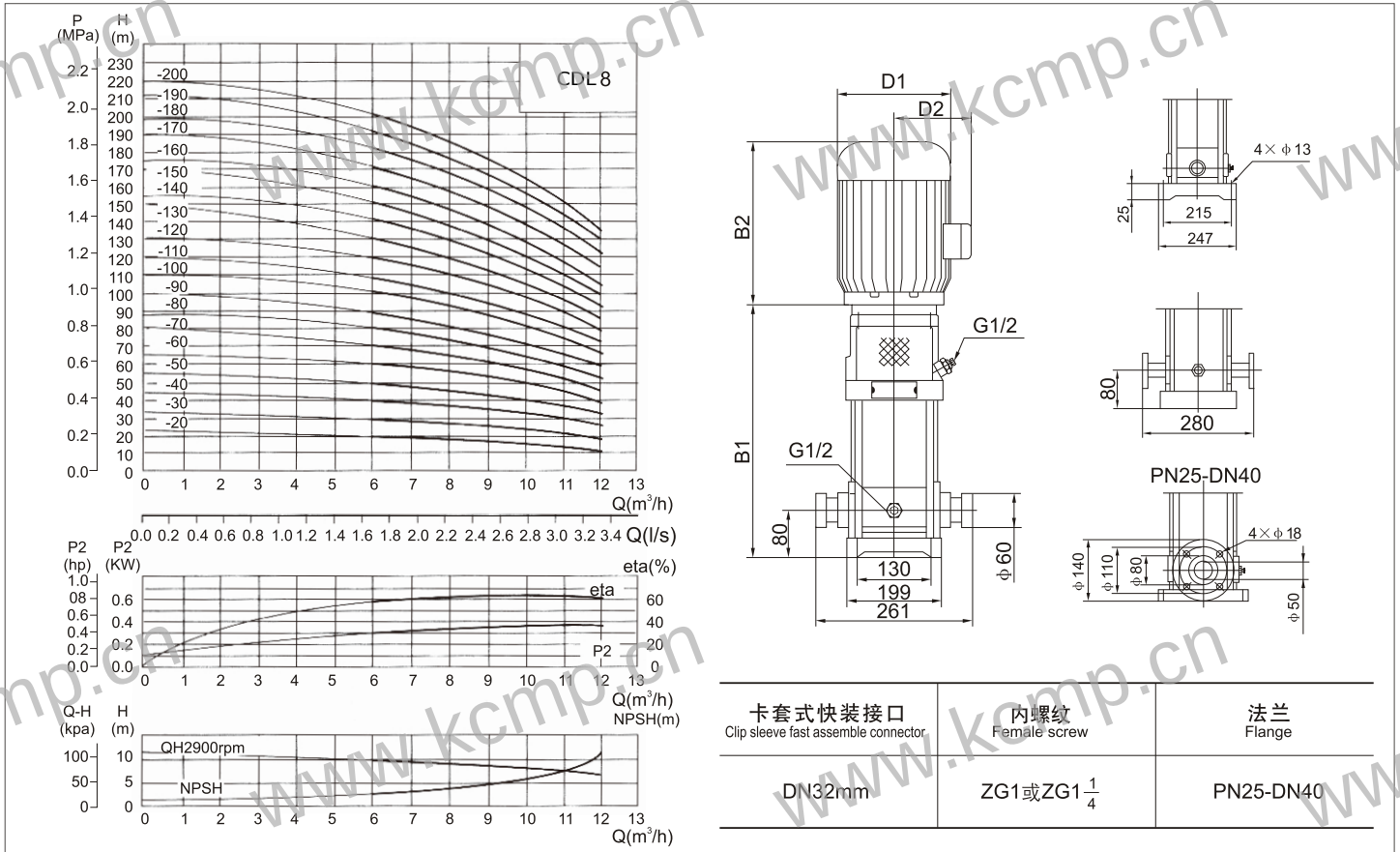
性能参数表及安装尺寸表 Performance Parameters and Installation Dimensions
