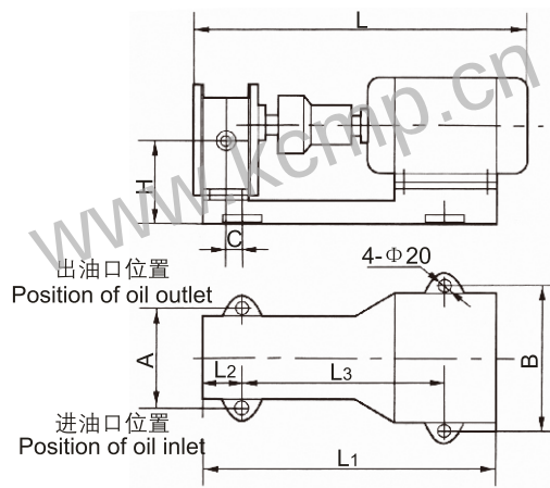
安装尺寸图 Installation Dimensions Drawing
